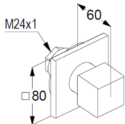
Maßzeichnung/ Dimensional drawing
