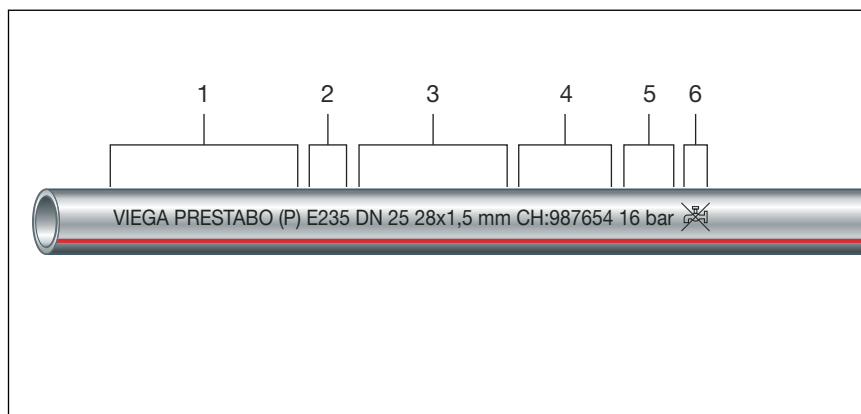
Abb. 8: Rohr innen und außen sendzimirverzinkt
