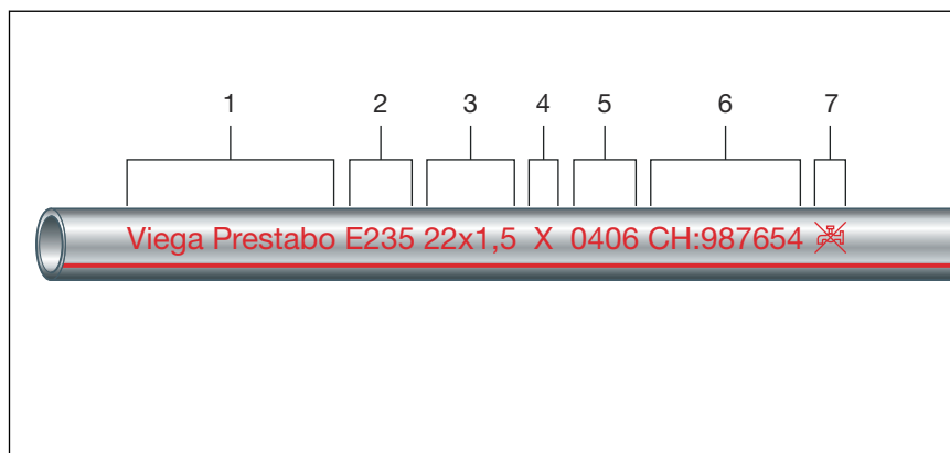
Abb. 6: Rohr galvanisch verzinkt
