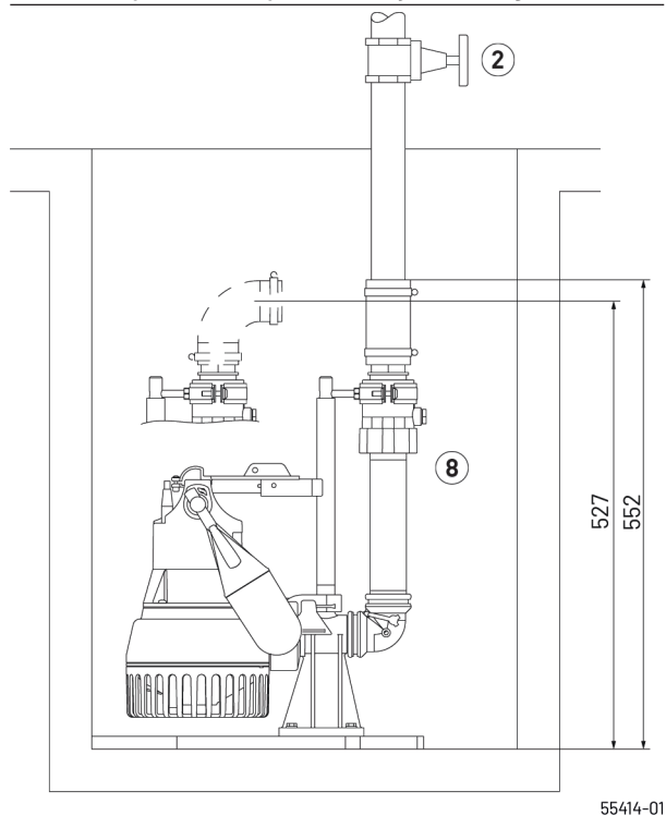
Einbaubeispiel und Hauptmaße Easyfix 32 Single
