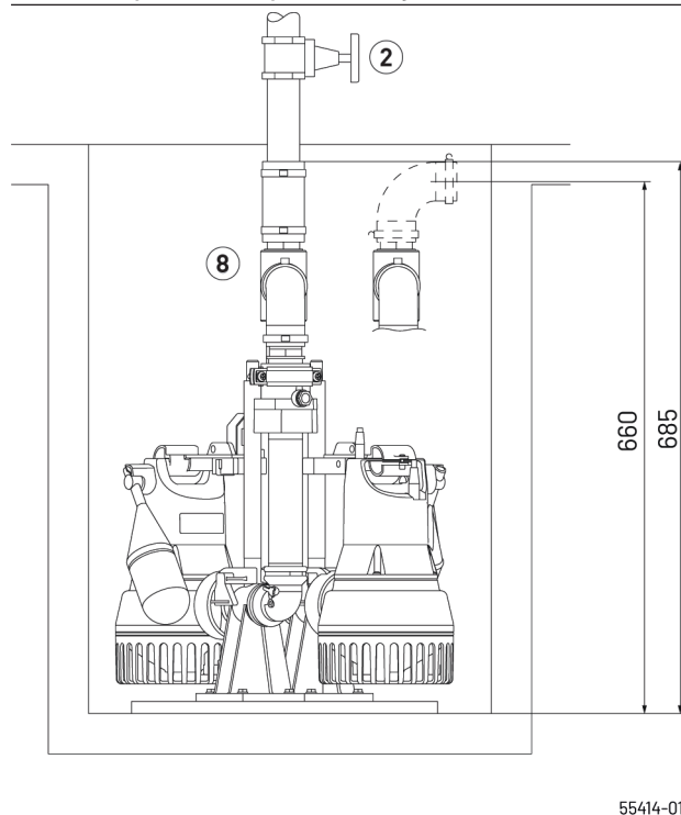
Einbaubeispiel und Hauptmaße Easyfix 32 Duo (mm)
