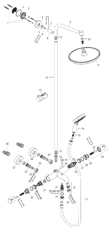
製品分解図
