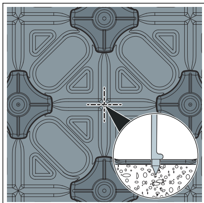
Abb. 3: Fonterra Base-Noppenplatte 15/17
