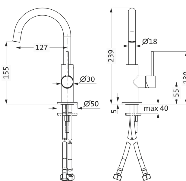
Lochbohrung 35mm
