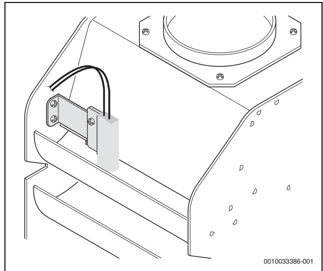
2 ZSR 5/11-5K
