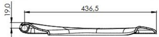
SCHNITT C-C
