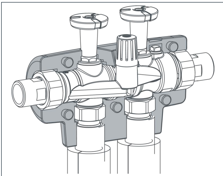
Abb. 4: Isolierschalen anbringen
