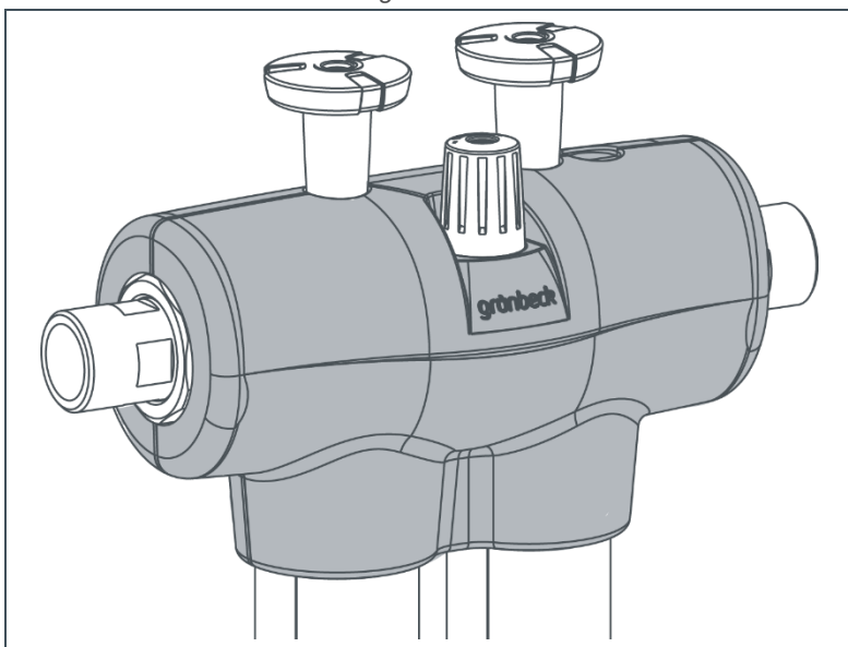
Abb. 5: Isolierschalen anbringen
