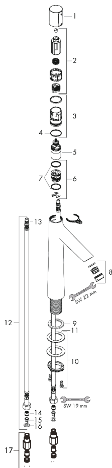
製品分解図
