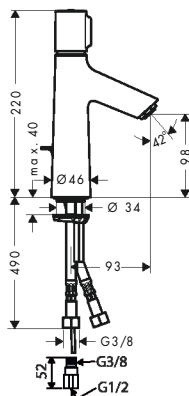
完成図
