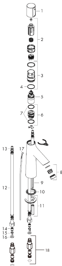
製品分解図
