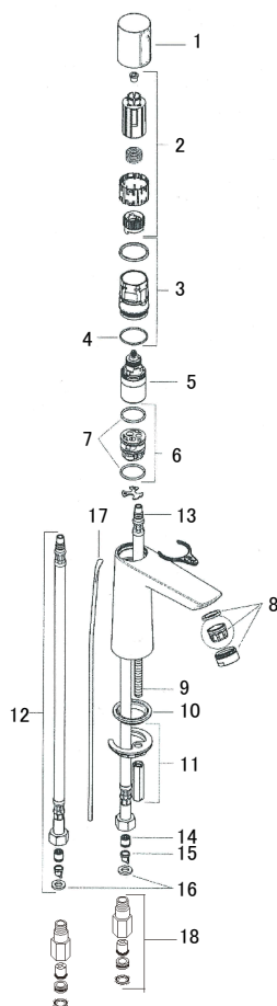
製品分解図
