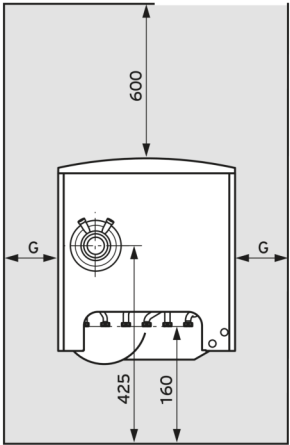
Draufsicht
